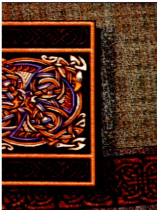
Billedet er taget fra disk 88, Charon
